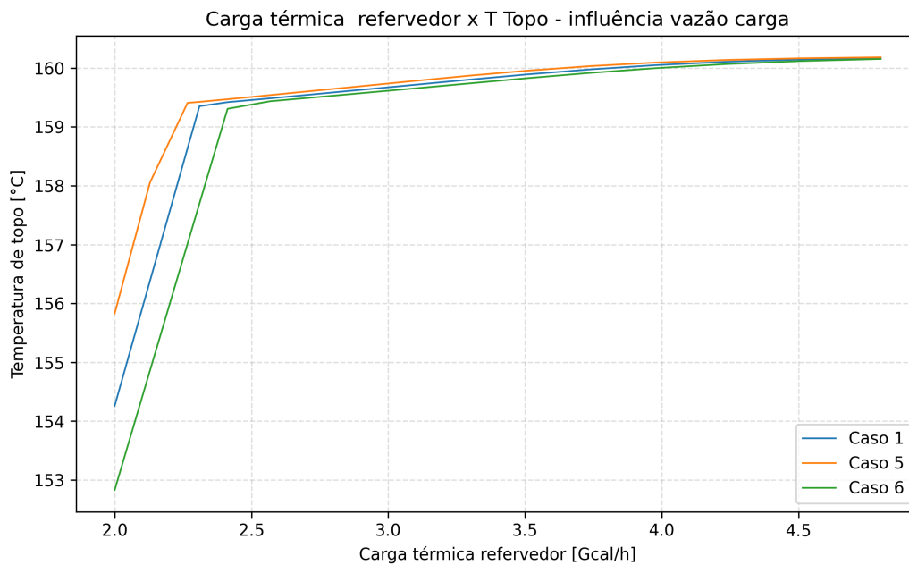
Figura 12: Carga térmica x temperatura do topo - Influência Vazão da Carga
