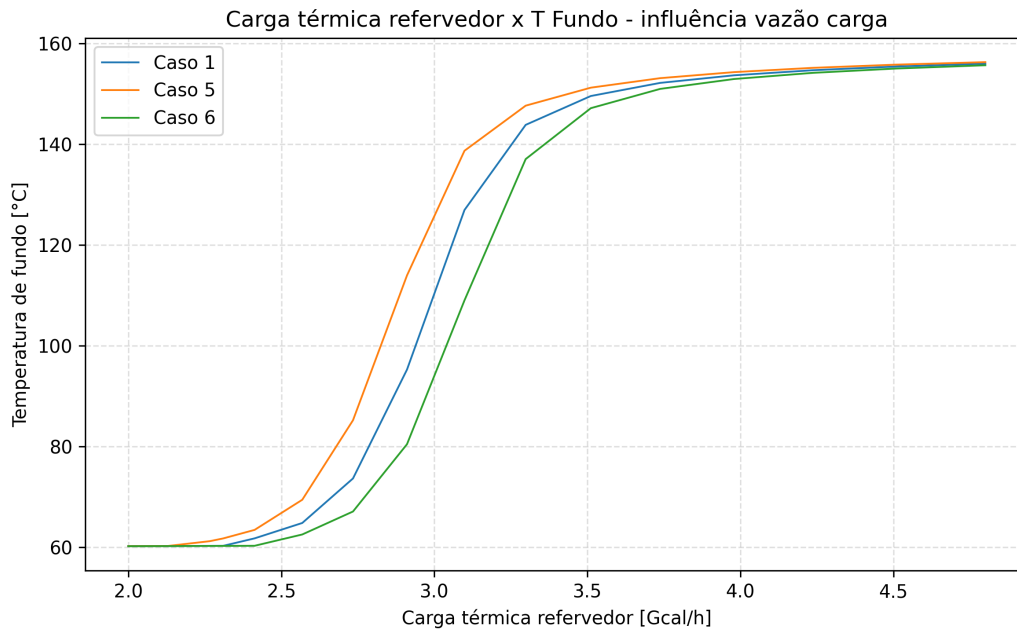
Figura 11: Carga térmica x temperatura do fundo - Influência Vazão da Carga
