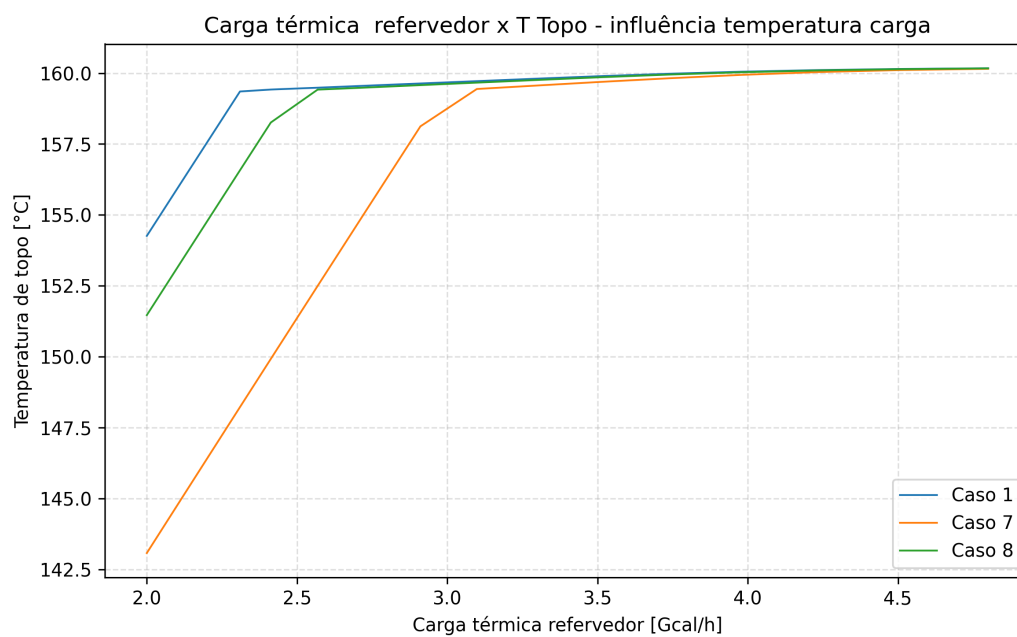
Figura 8: Carga térmica x temperatura do topo - Influência Temperatura da Carga
