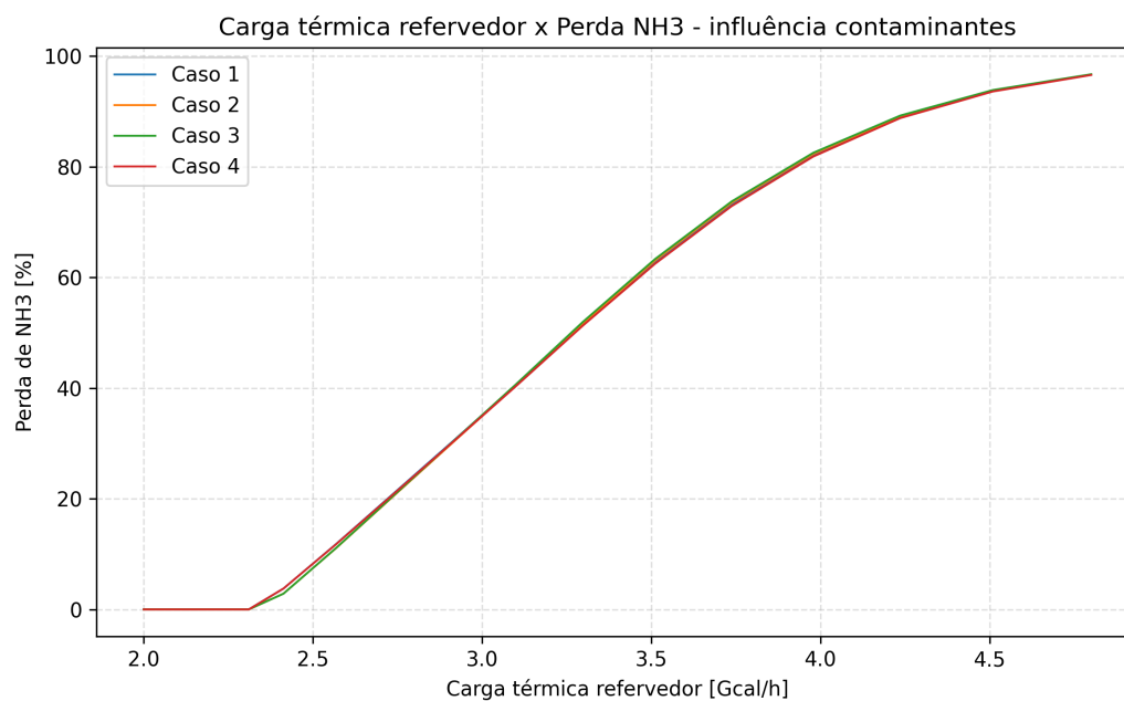
Figura 2: Carga térmica x perda de NH 3 - Influência Contaminantes
