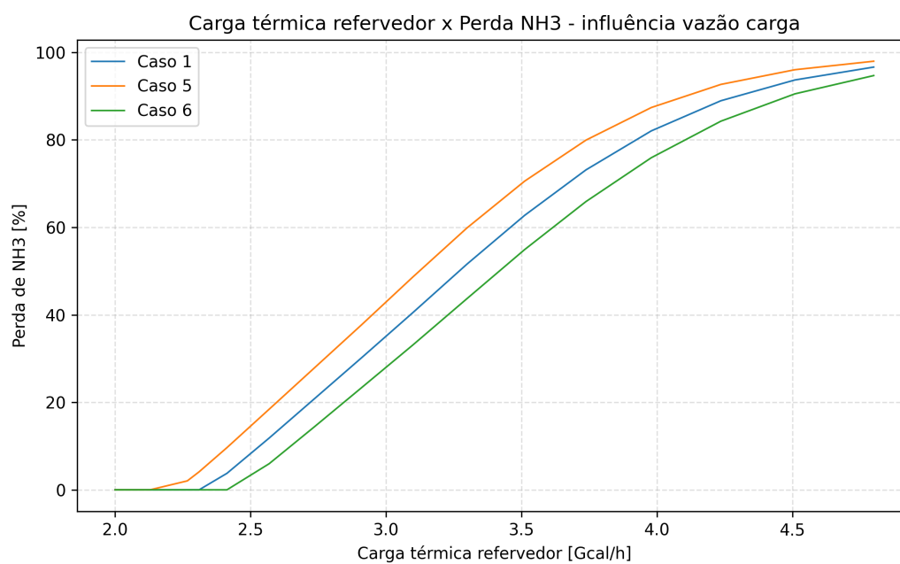
Figura 10: Carga térmica x perda de NH 3 - Influência Vazão da Carga
