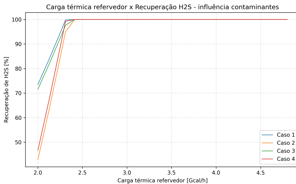
Figura 1: Carga térmica x recuperação de H 2 S - Influência Contaminantes
