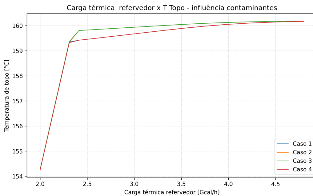
Figura 4: Carga térmica x temperatura do topo - Influência Contaminantes
