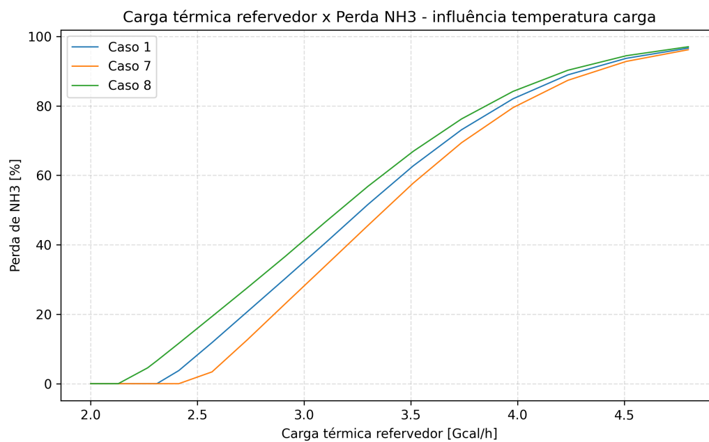
Figura 6: Carga térmica x perda de NH 3 - Influência Temperatura da Carga
